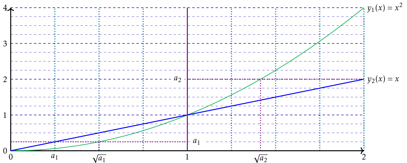
FIGURE 1 – Fonctions y_1(x) = x^2 et y_2(x) = x
