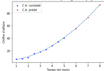
Prédiction du chiffre d'affaire par régression polynômiale
