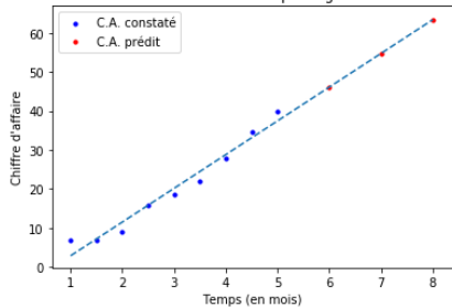
Prédiction du chiffre d'affaire par régression linéaire
