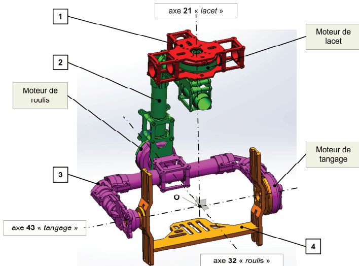
Fig.2, vue de la nacelle seule
